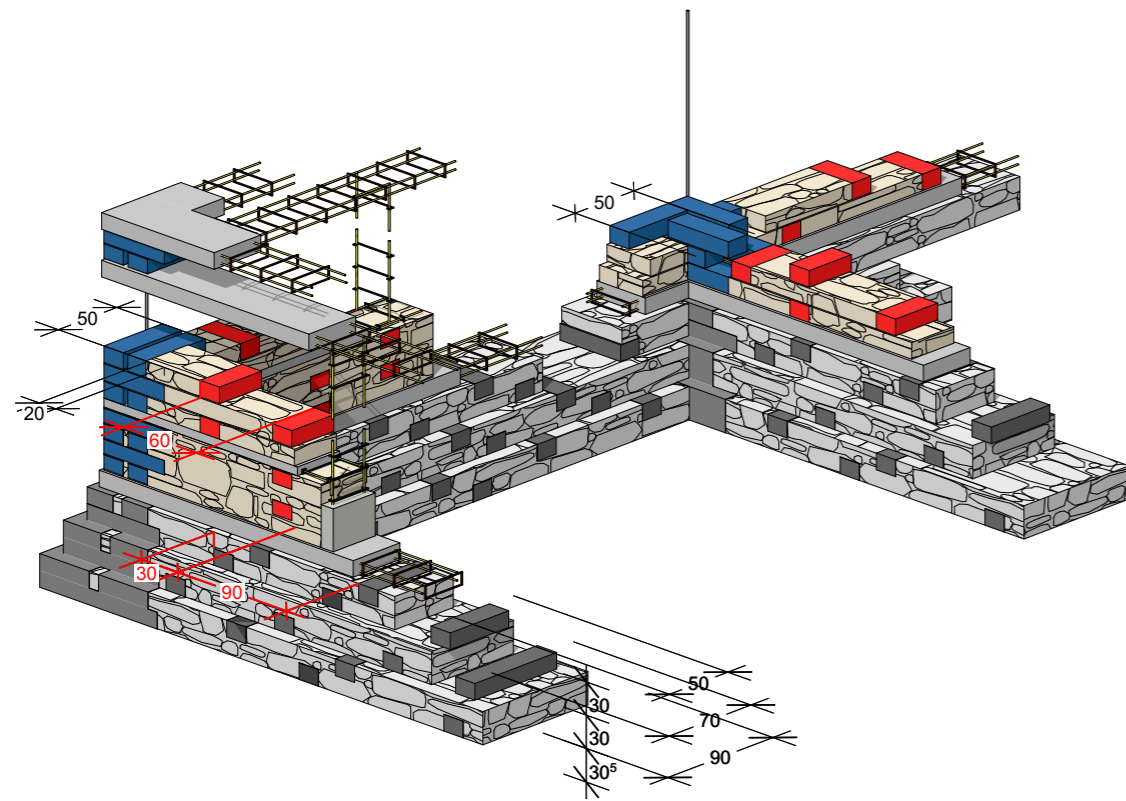
VUE AXONOMETRIQUE FONDATION
