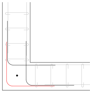
PLIAGE DE FER À BÉTON
