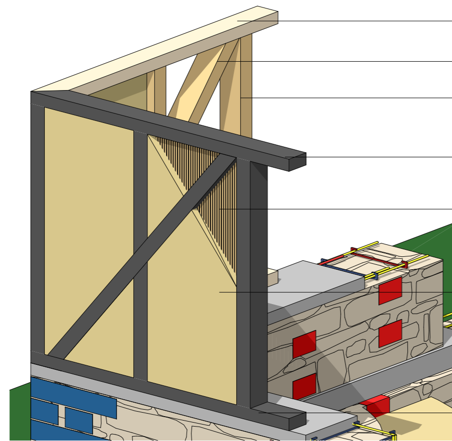
VUE AXONOMETRIQUE FONDATION
