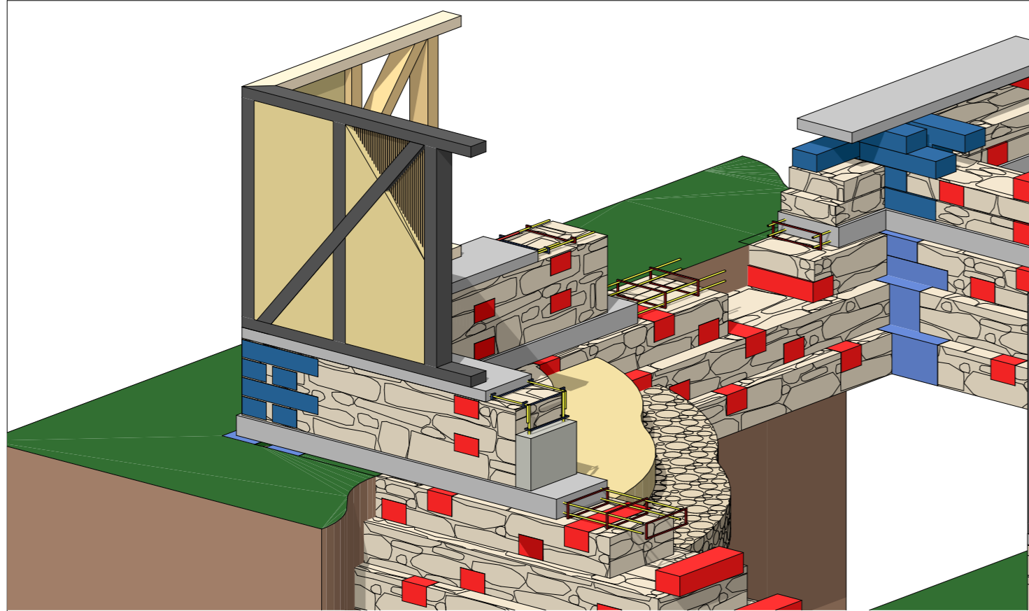
VUE AXONOMETRIQUE GENERALE
